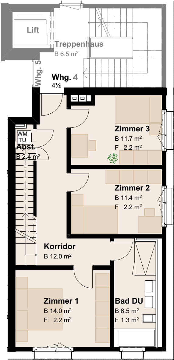
2.Obergeschoss
